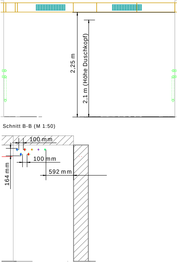
Schnitt C-C (M 1:50)
