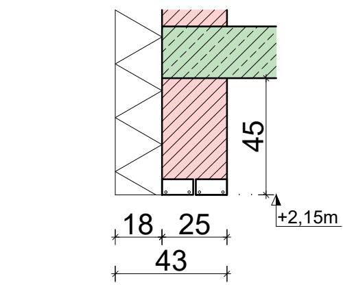
Sturz Hauseingangstür
