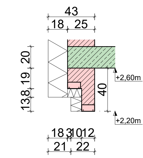
Fenstersturz Rollo bis 2,00m Spannweite
