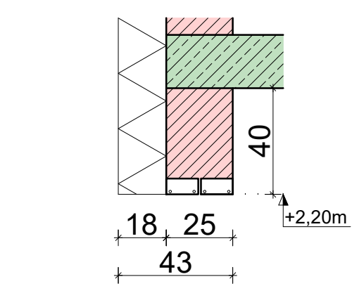
Fenstersturz ohne Rollo
