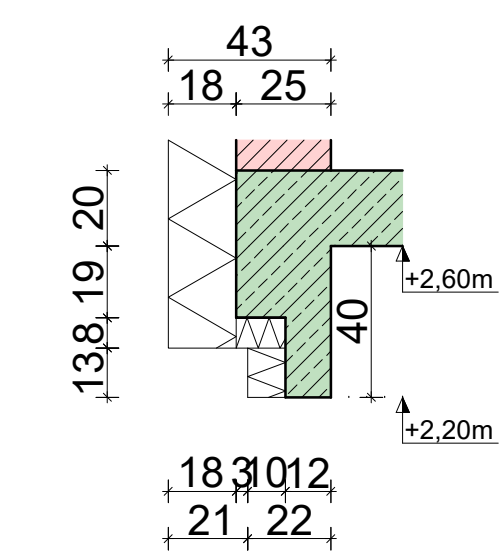
Fenstersturz Rollo ab 2,00m Spannweite
