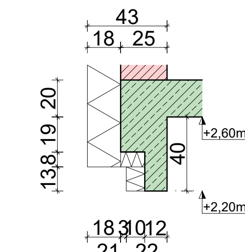
Fenstersturz Rollo ab 2,00m Spannweite + grüne Markierung beachten!!!
