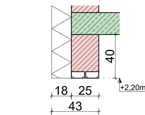
Fenstersturz ohne Rollo
