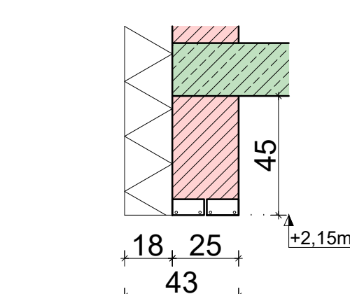
Sturz Hauseingangstür
