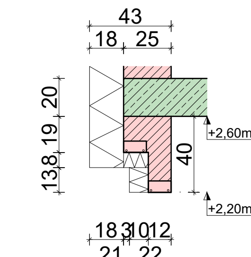
Fenstersturz Rollo bis 2,00m Spannweite
