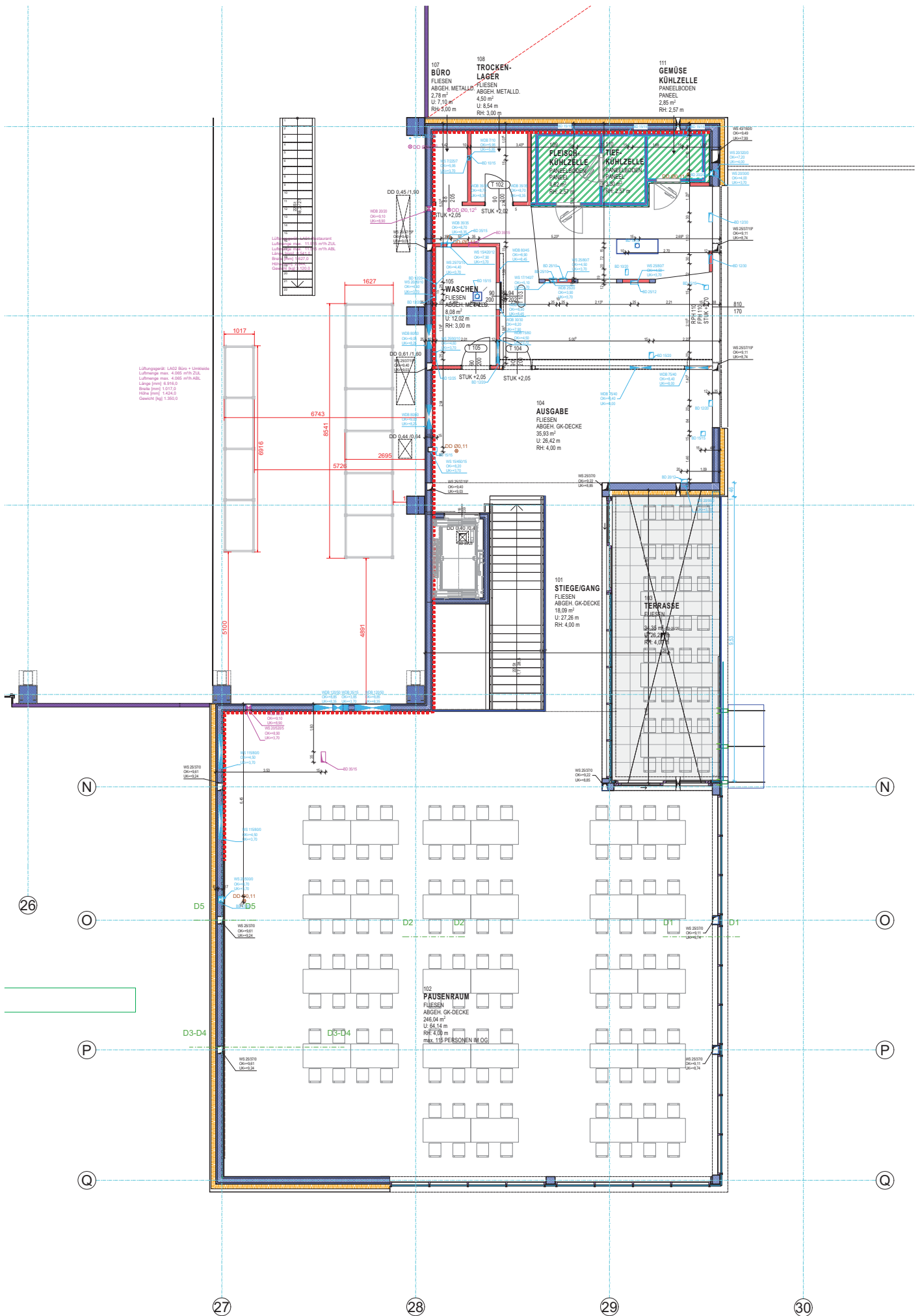
BRANDABSCHOTTUNGEN OBERGESCHOSS - M=1:100
