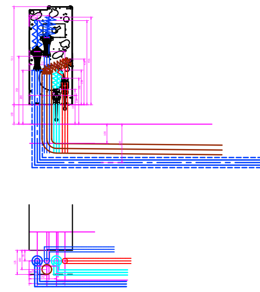
M1:20
