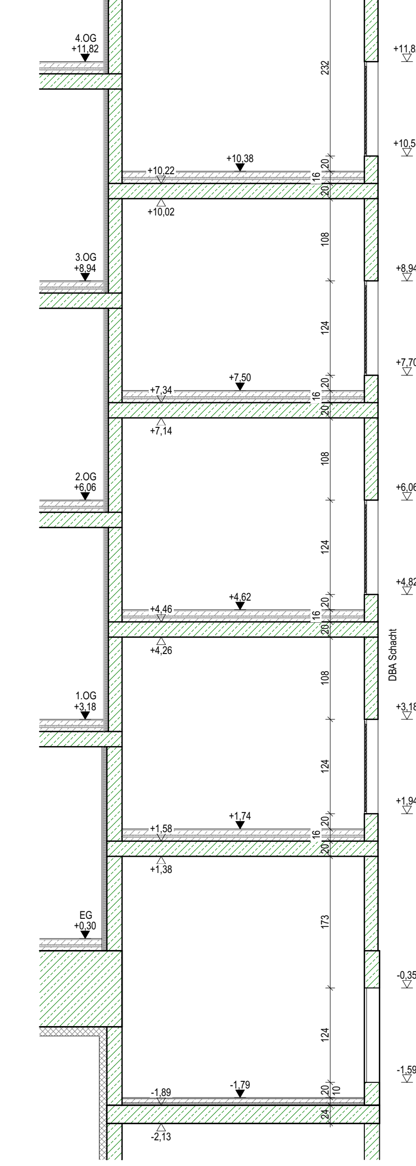
Hilfsschnitt X-X
