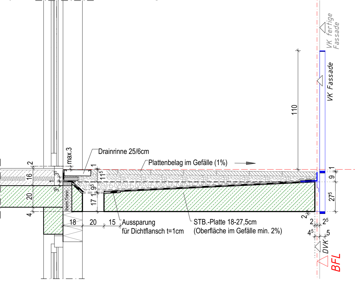
Systemschnitt Entwässerung:
