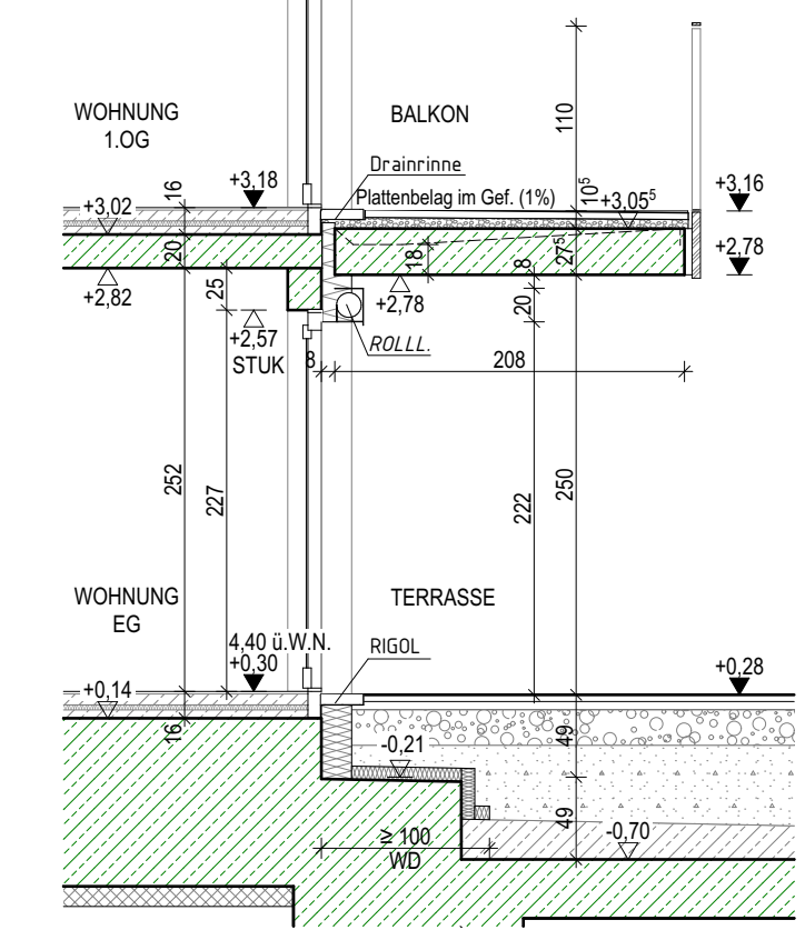
K2-K2
