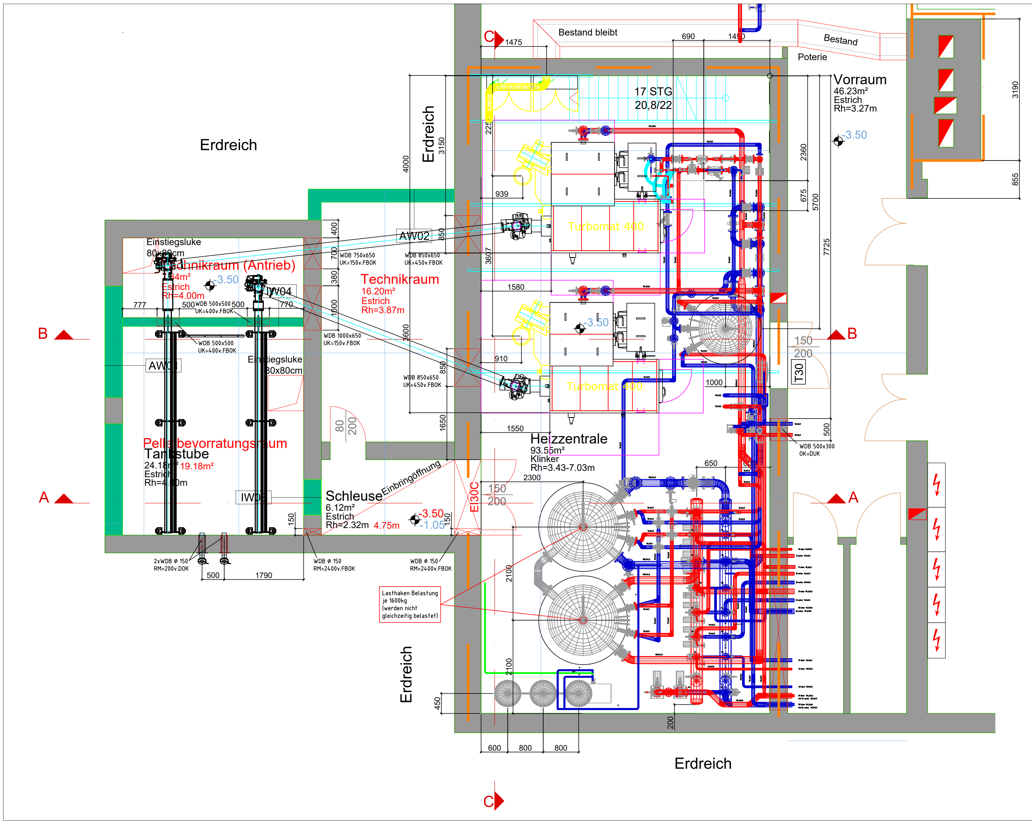
GRUNDRISS
