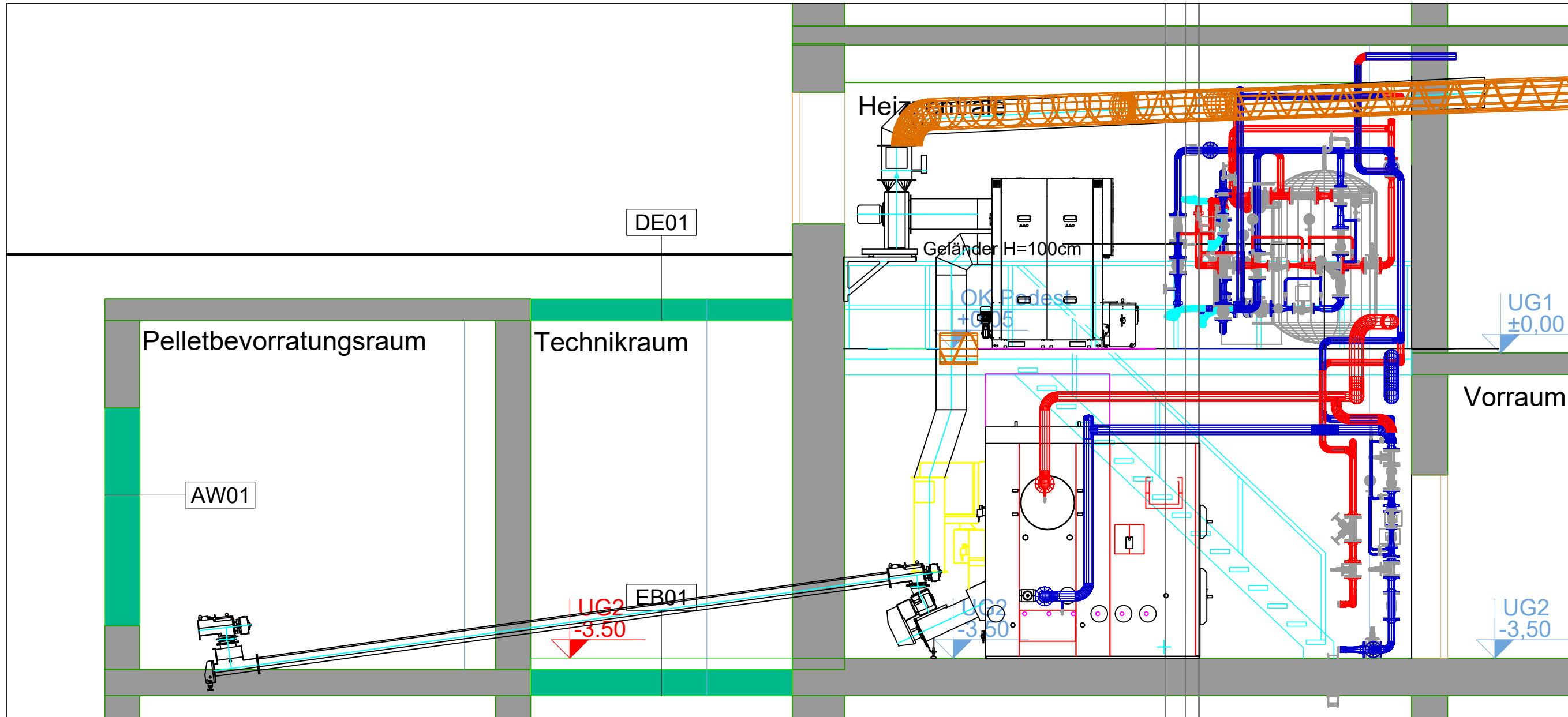
SCHNITT C-C
