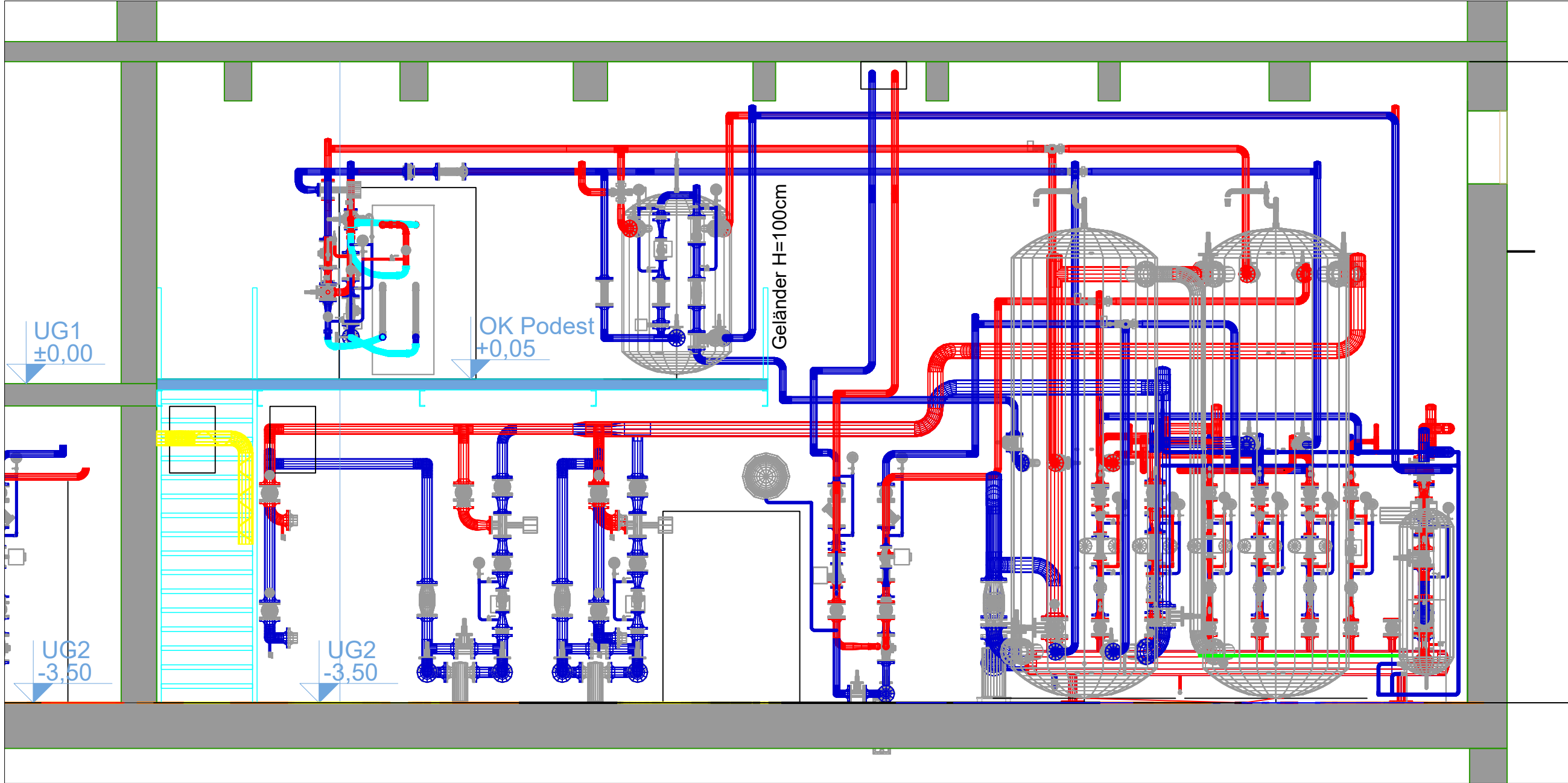
SCHNITT C-C
