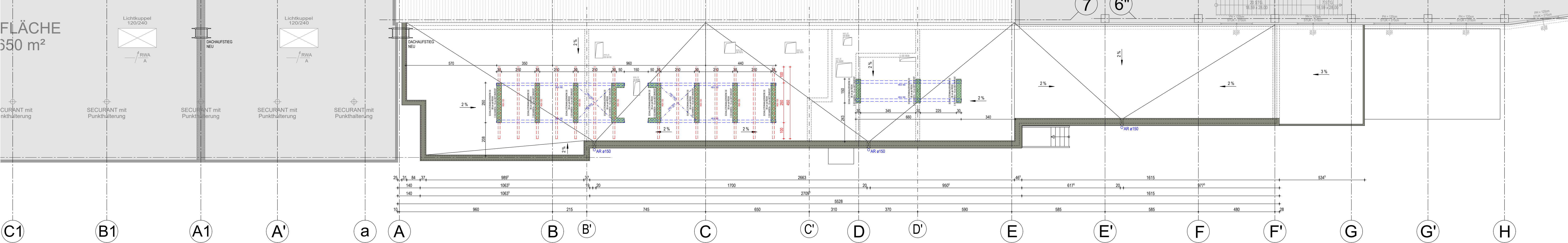
Grundriss DACHDRAUFSICHT Trakt "A" M 1:100
