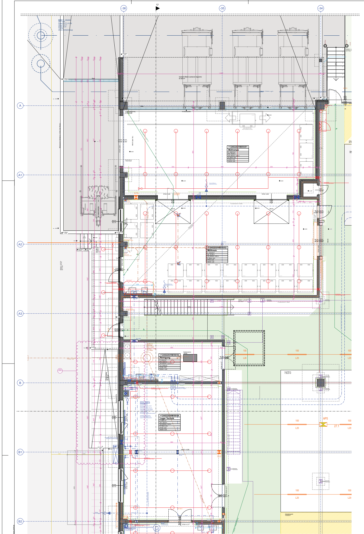
Grundriss Erdgeschoß Halle Müll | 1:50
