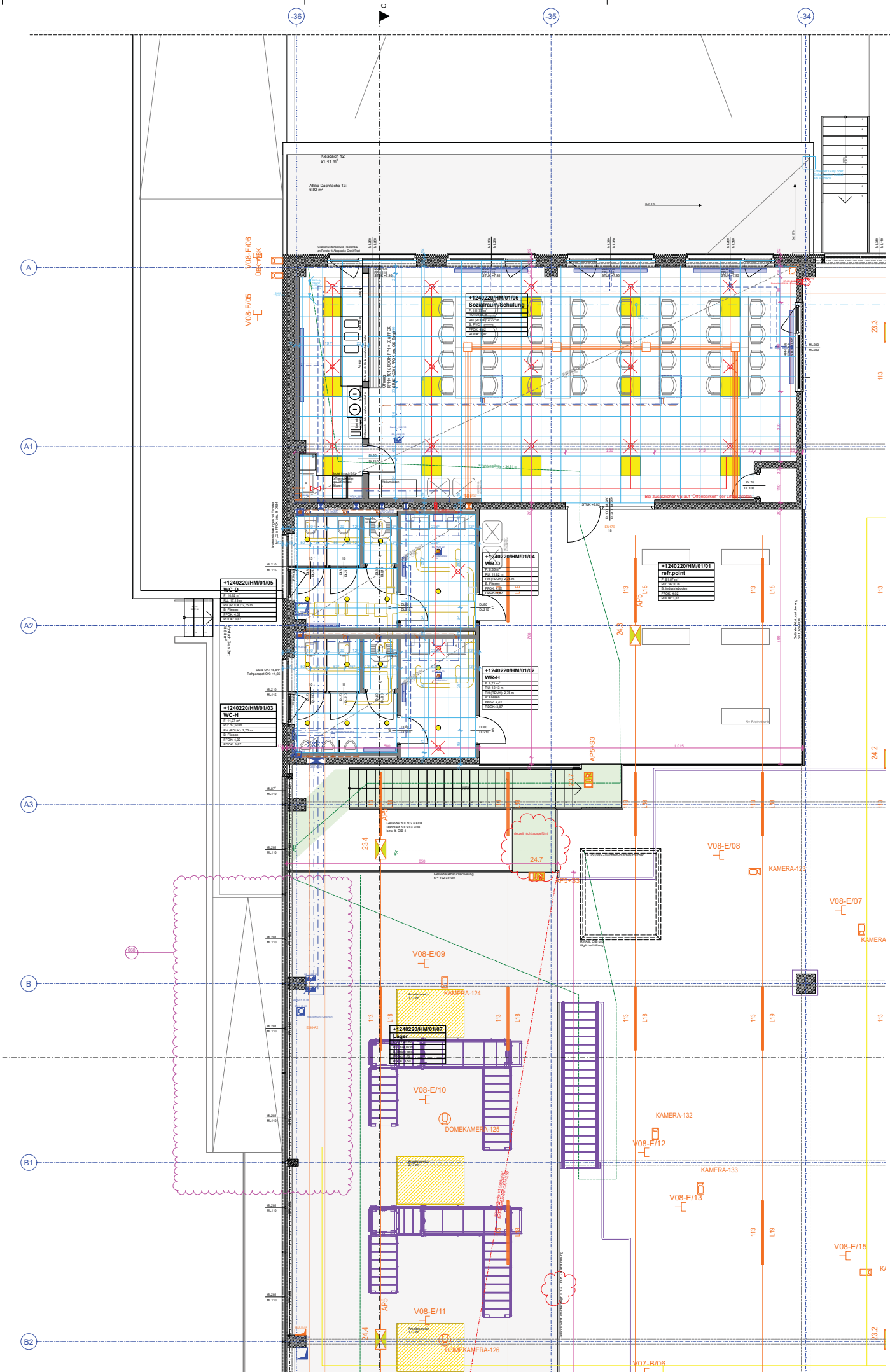
Grundriss 1. Obergeschoß Halle Müll | 1:50
