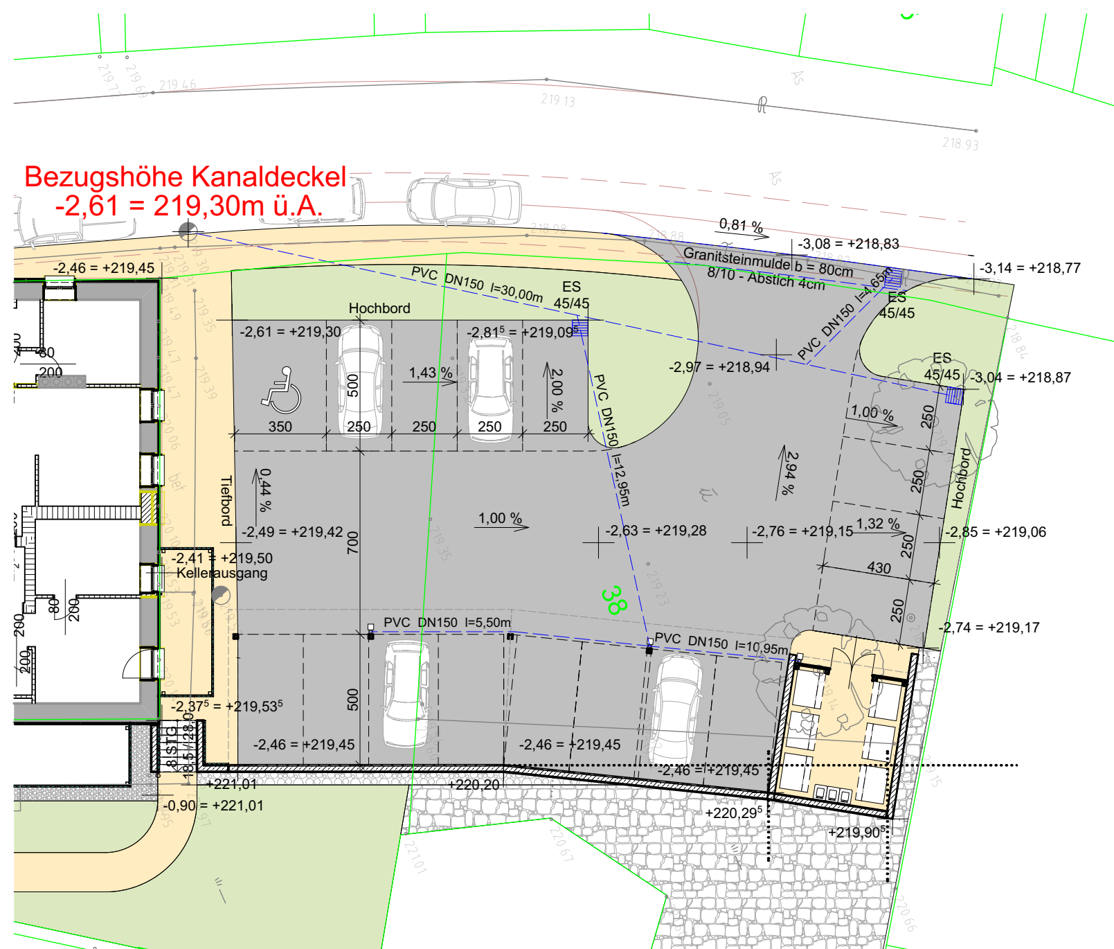
LAGEPLAN 1:200
