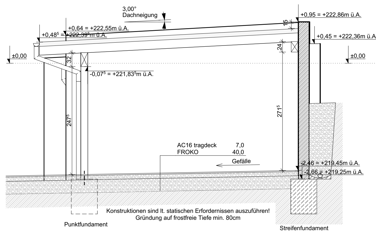
SCHNITT C1-C1
