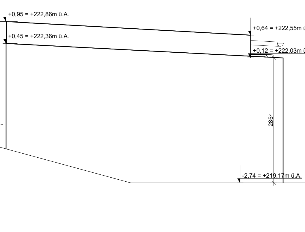
ANSICHT NORD-OST
