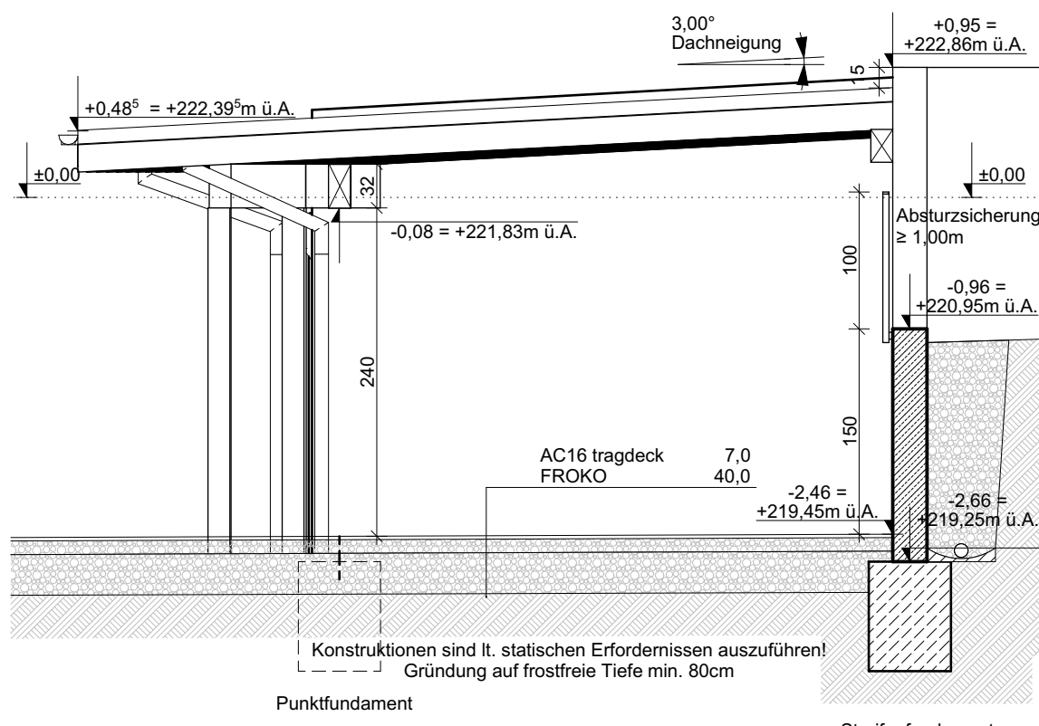
SCHNITT C2-C2
