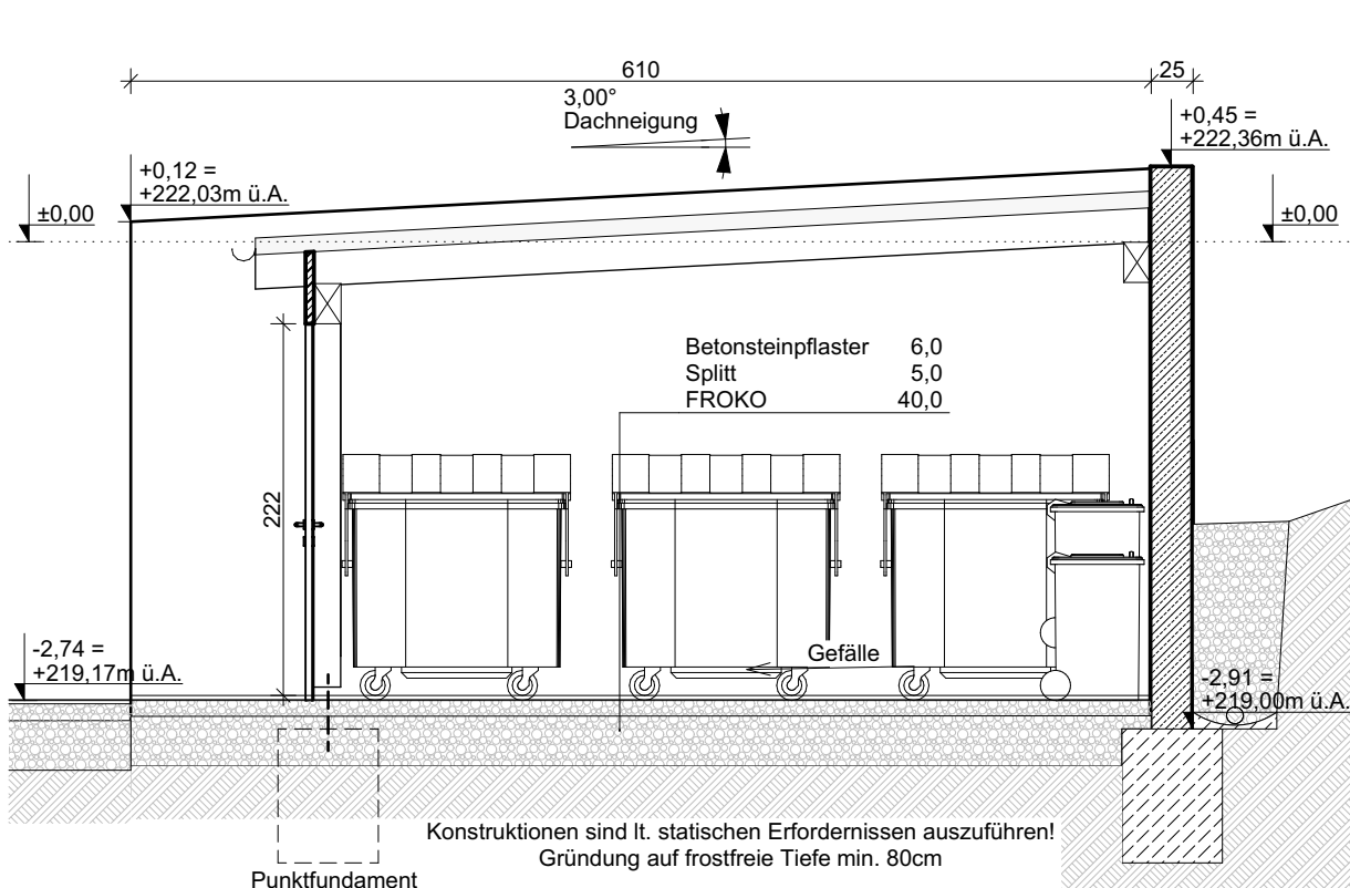
SCHNITT C3-C3
